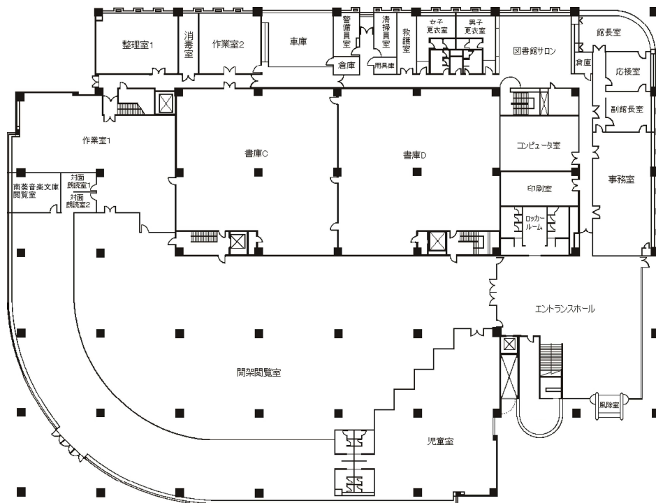
1 F 平面図
