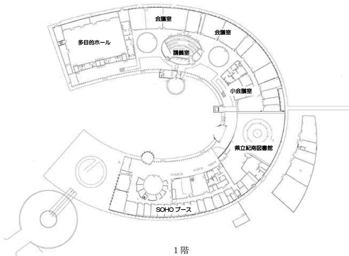
県立情報交流センターBig・U 平面図
